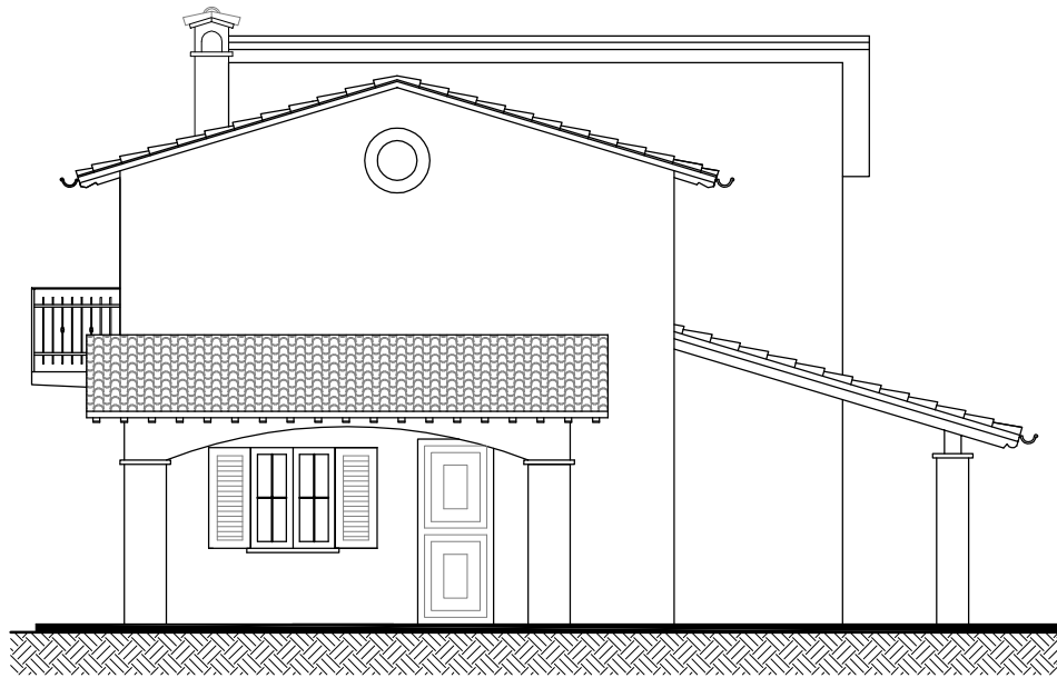
PROSPETTO NORD-EST
