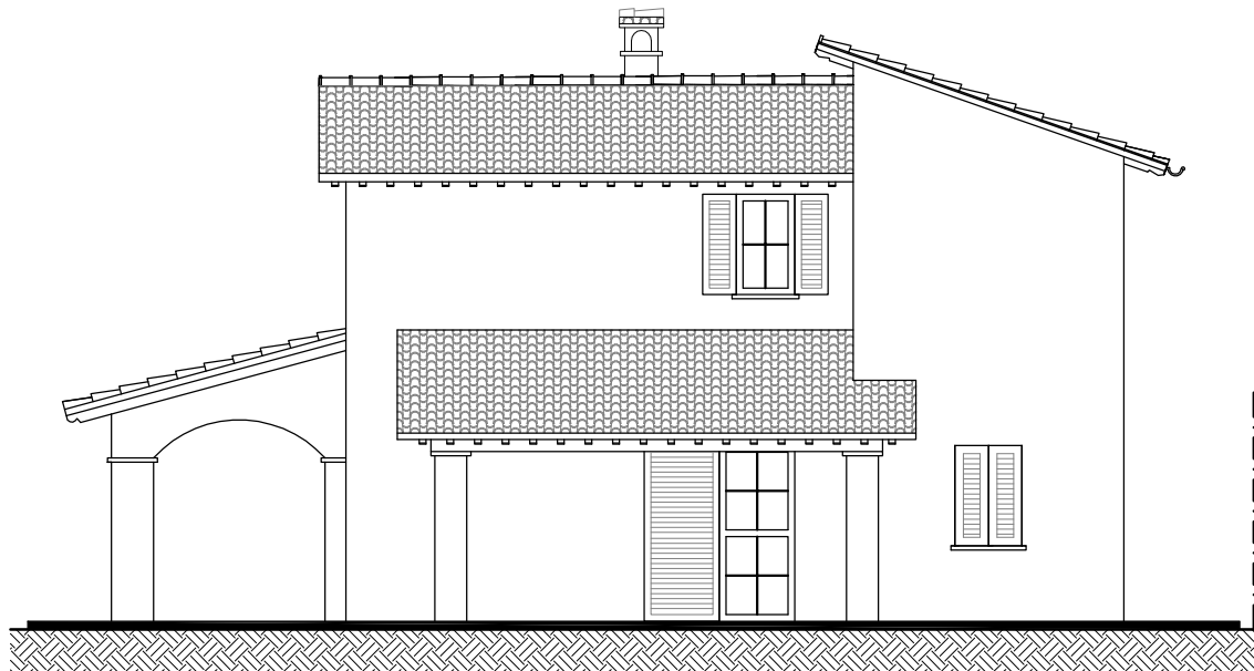
PROSPETTO NORD-OVEST
