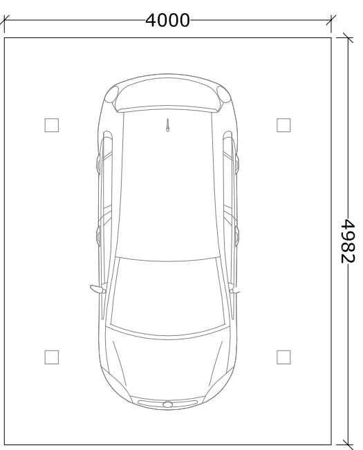
INGOMBRO COPERTURA
